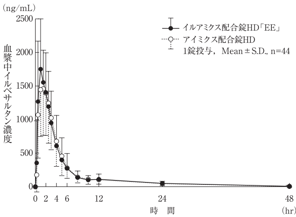
血漿中イルベサルタン濃度推移
