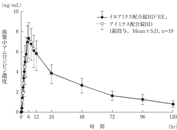
血漿中アムロジピン濃度推移
