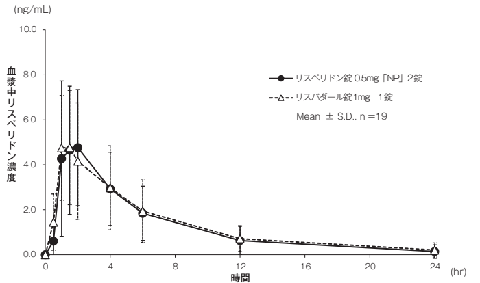
血漿中リスペリドン濃度推移
