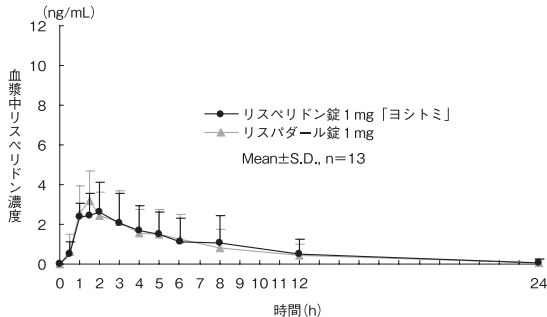
血漿中リスベリドン濃度推移
