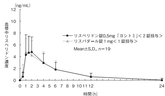
血漿中リスペリドン濃度推移
